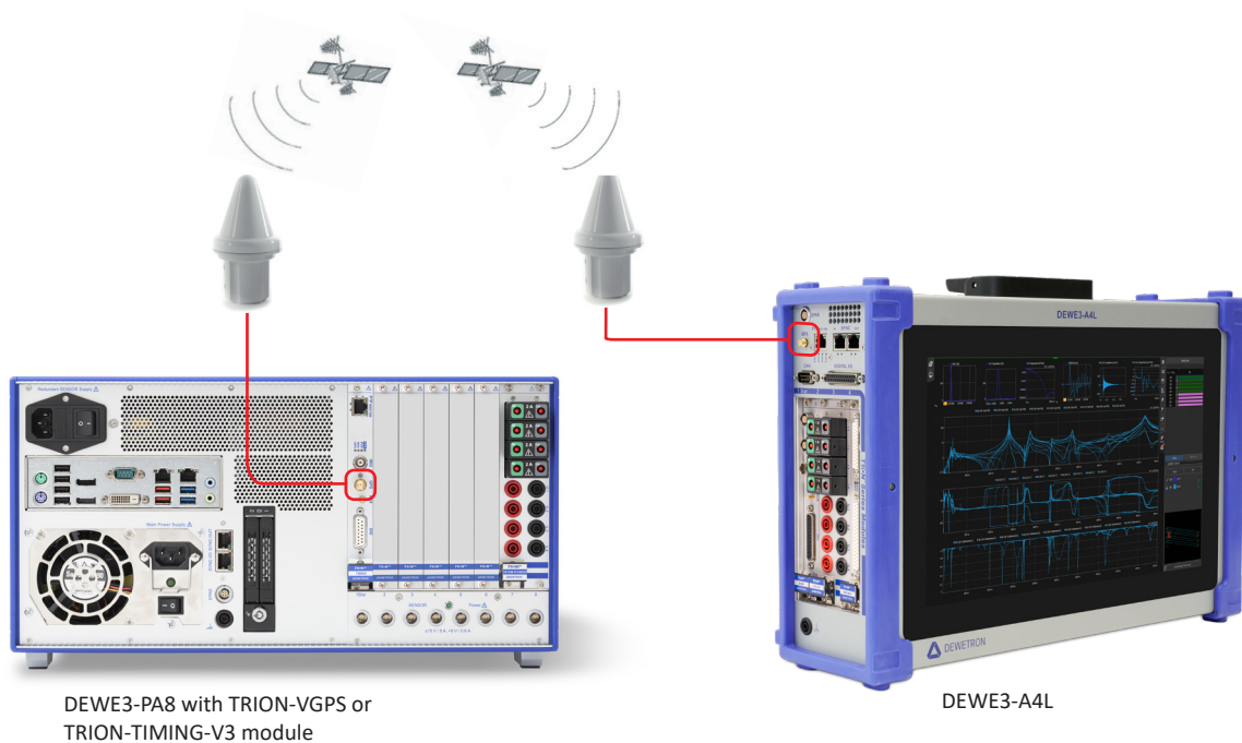
Fig. 31: GPS sync
