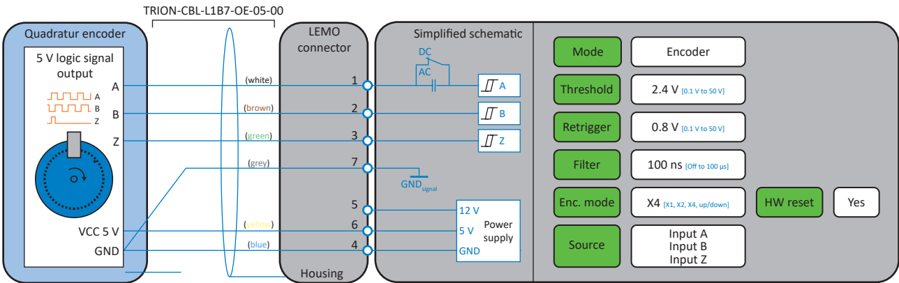
Fig. 199: Quadratur encoder
