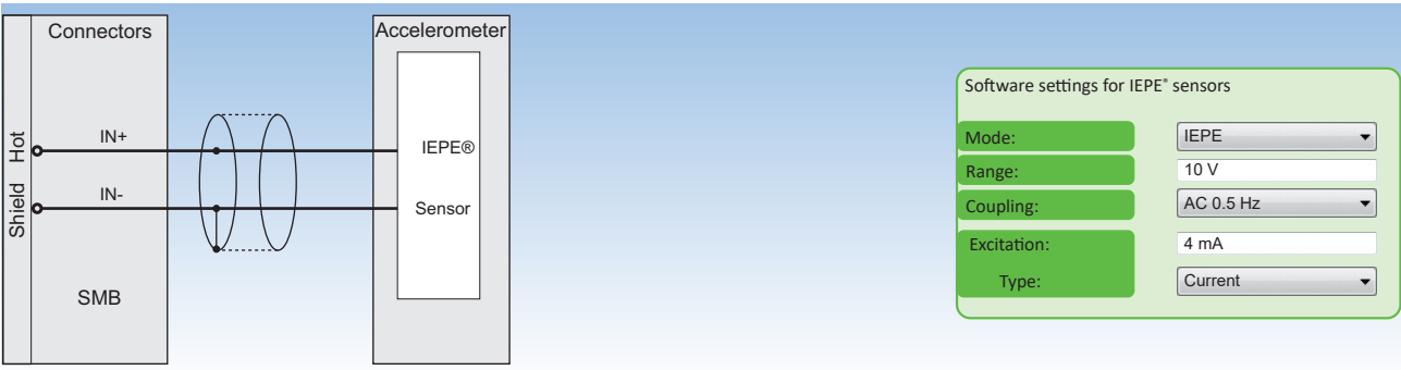
Fig. 140: IEPE® sensor
