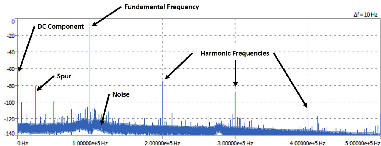
Fig. 234: FFT chart of TRION-1620-ACC
