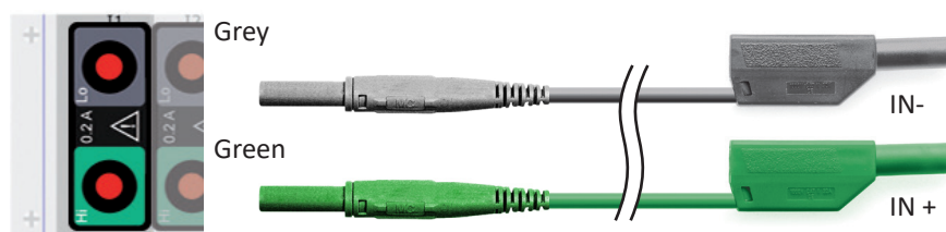
Fig. 145: Current input module
