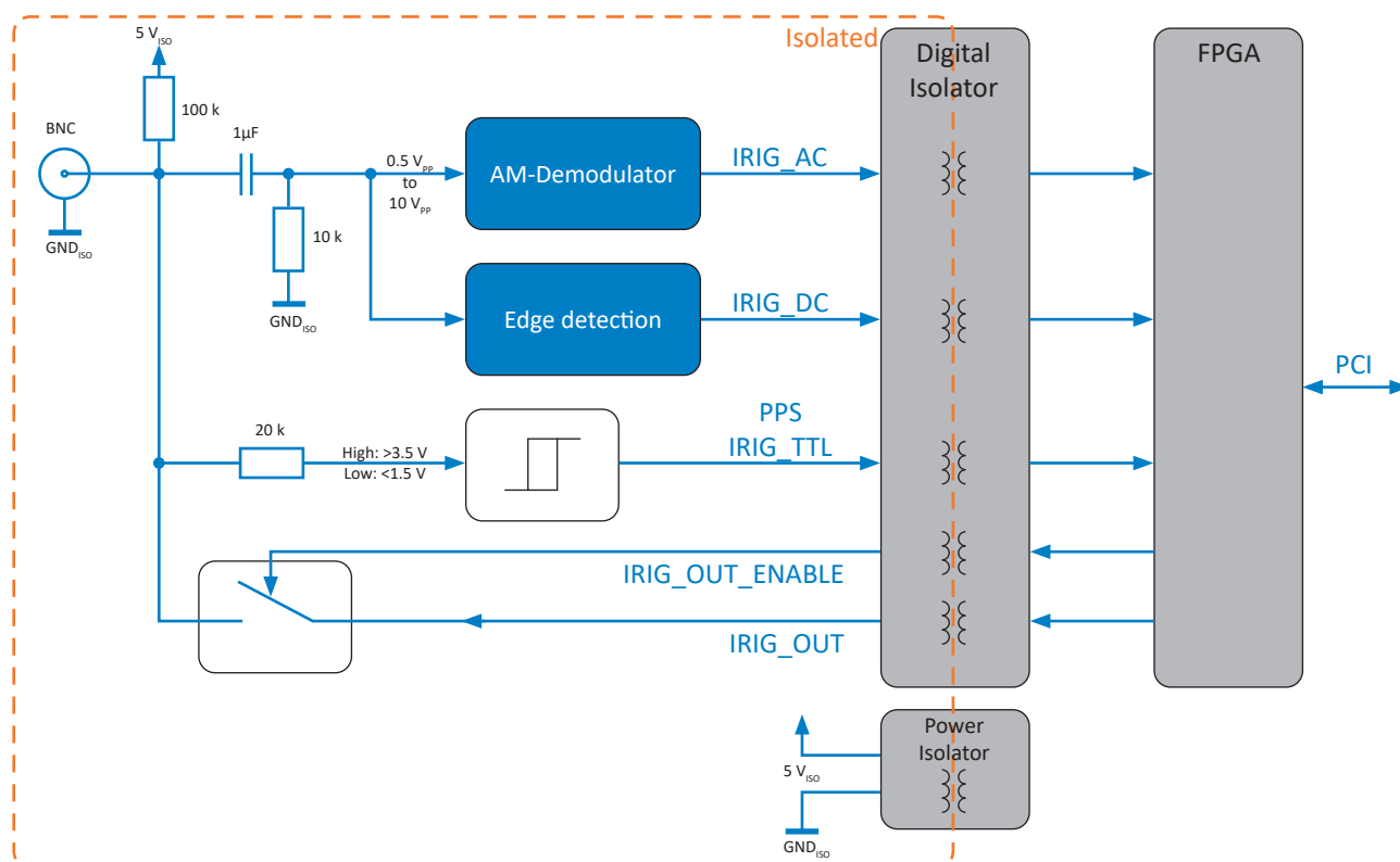
Fig. 184: BNC (IRIG) input
