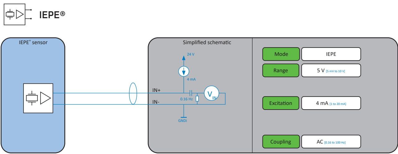
Fig. 87: IEPE® sensor
