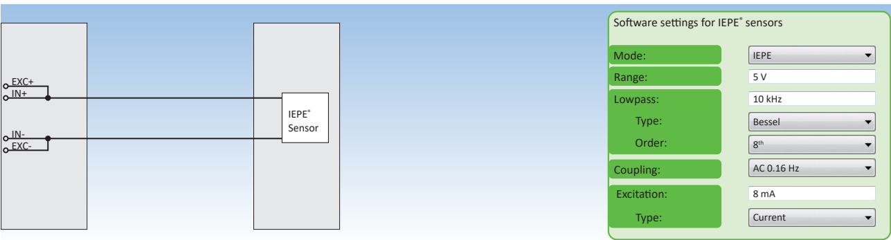
Fig. 60: IEPE® sensor
