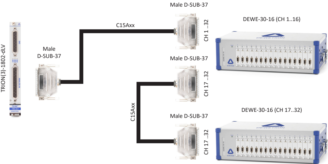
Fig. 233: C15Axx overview
