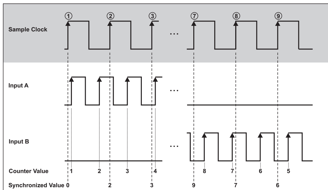
Fig. 215: A-Up/B-down encoder
