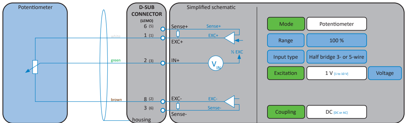
Fig. 51: Potentiometer
